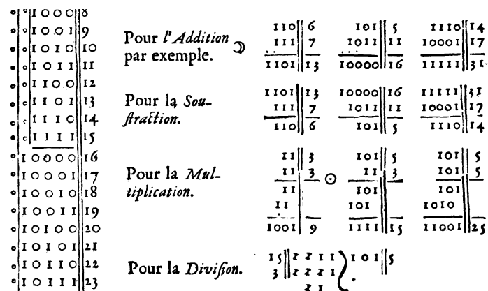
Abbildung 2: Rechnen im Dualsystem nach Leibniz 1705 (aus [Ro92])
